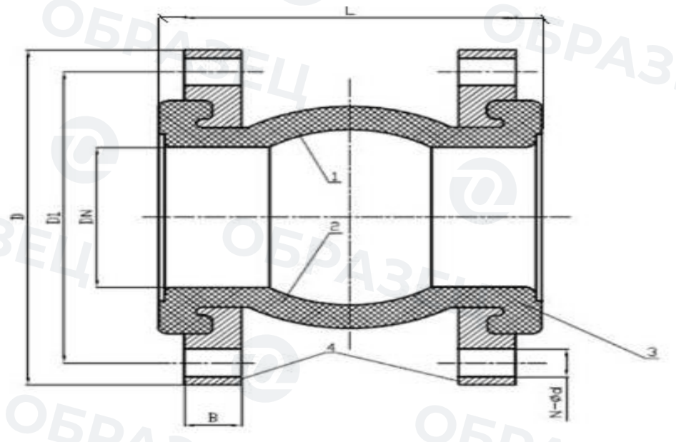
Рисунок 1 - Компенсатор резиновый фланцевый
