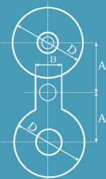
Рисунок 2 – Заглушка поворотная плоская Т-ММ-25-01-06, где D – диаметр, A – межосевое расстояние м/у заглушкой и кольцом, B – ширина вставки DN: 25, 50–150 PN: от 0,6 до 10,0 МПа T: от минус 70 до 450 °С Сталь: 20, 09Г2С, 12Х18Н10Т, 13ХФА и др.
