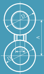
Рисунок 1 – Заглушка поворотная стальная для фланцев арматуры АТК 26-18-5-93, где D – диаметр, A – межосевое расстояние м/у заглушкой и кольцом, B – осевое расстояние м/у вставками DN: 25, 50–150 PN: от 1,6 до 16,0 МПа T: от минус 70 до 475 °С Сталь: 20, 09Г2С, 12Х18Н10Т, 13ХФА и др.
